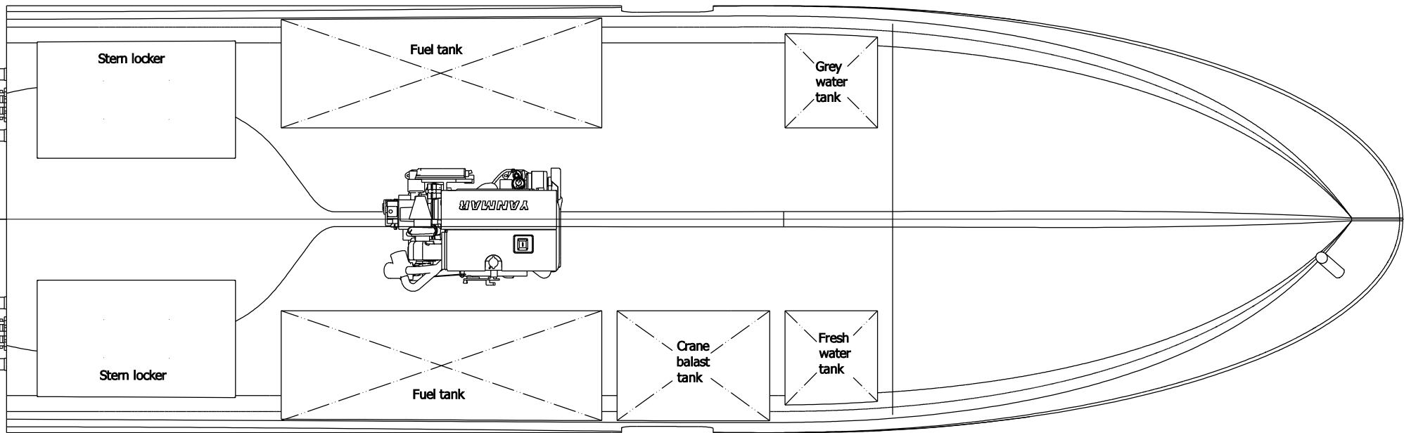
Tank plan (Plan zbiorników)
