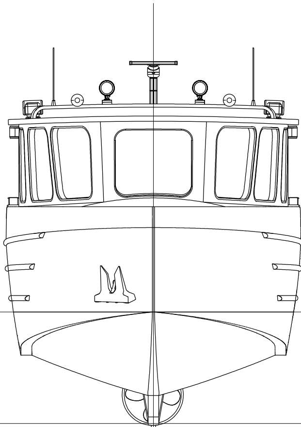
Bow view (Widok od dziobu)
